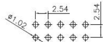
P.C.B Hole Layout
