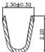
SEC A-A
