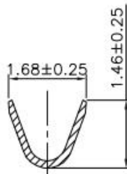
SEC:A-A
