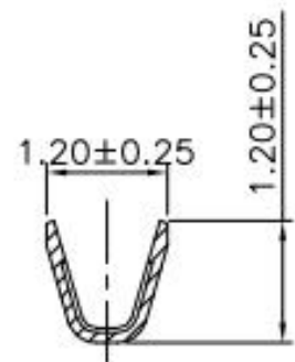
SEC:B-B
