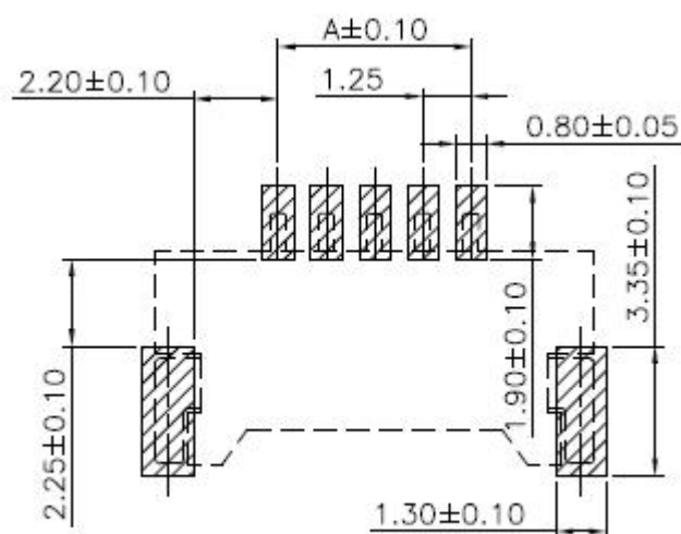
P.C.B. LAYOUT
