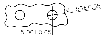
P.C.Board Hole Pattern
