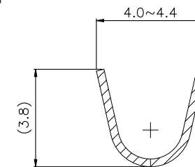
Section D-D
