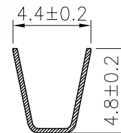
SEC A-A
