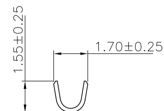
SEC:B-B
