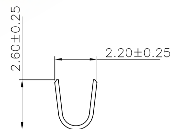
SEC:A-A
