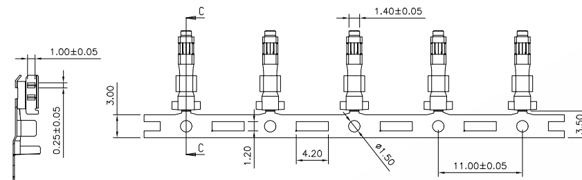
SLICE C-C
