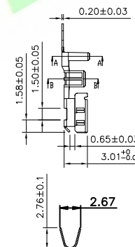
SLICE B-B
