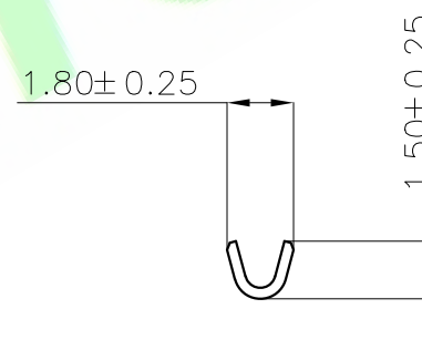
SEC:B-B
