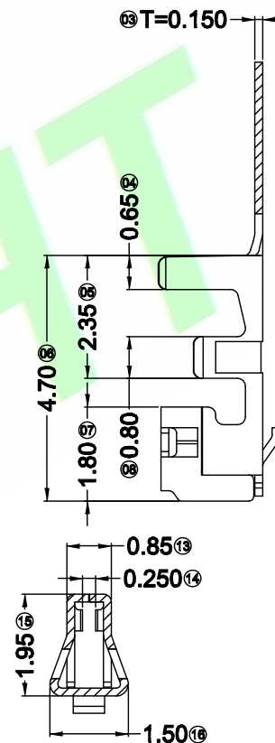
SECTION: C-C SCALE: 1:1
