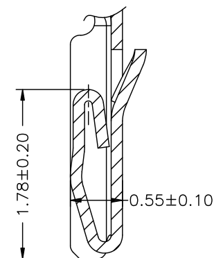
SEC:D-D
