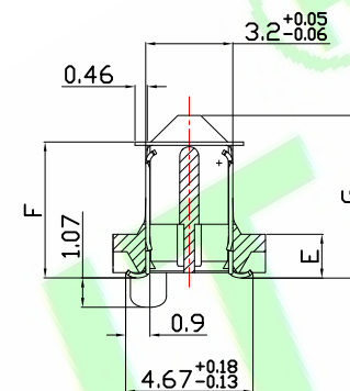
SECTION A-A SCALE 2:1
