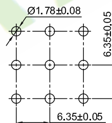
P.C.B LAYOUT
