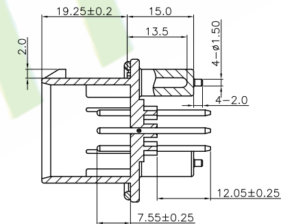
SEC A-A
