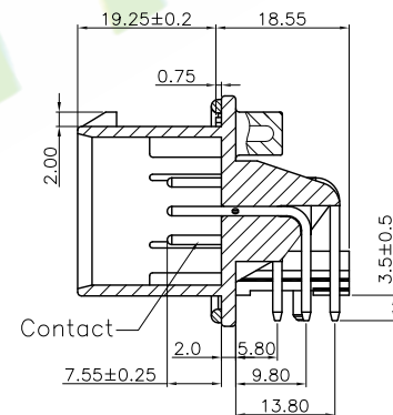
SEC A-A
