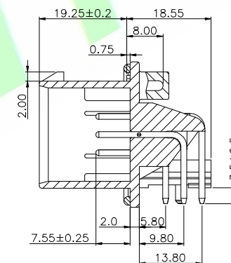
SEC A-A
