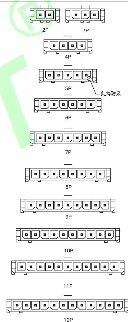
PH3.0 Wafer 防呆位置分部示意图
