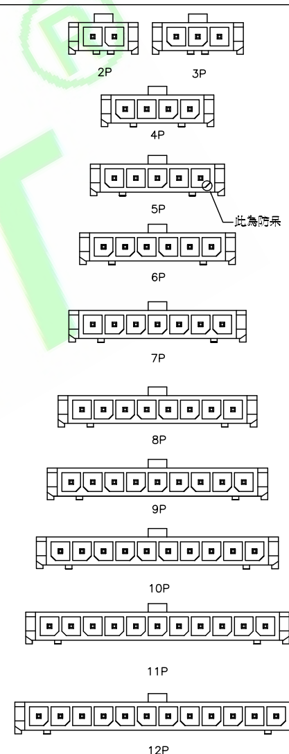
PH3.0 Wafer 防呆位置分部示意图
