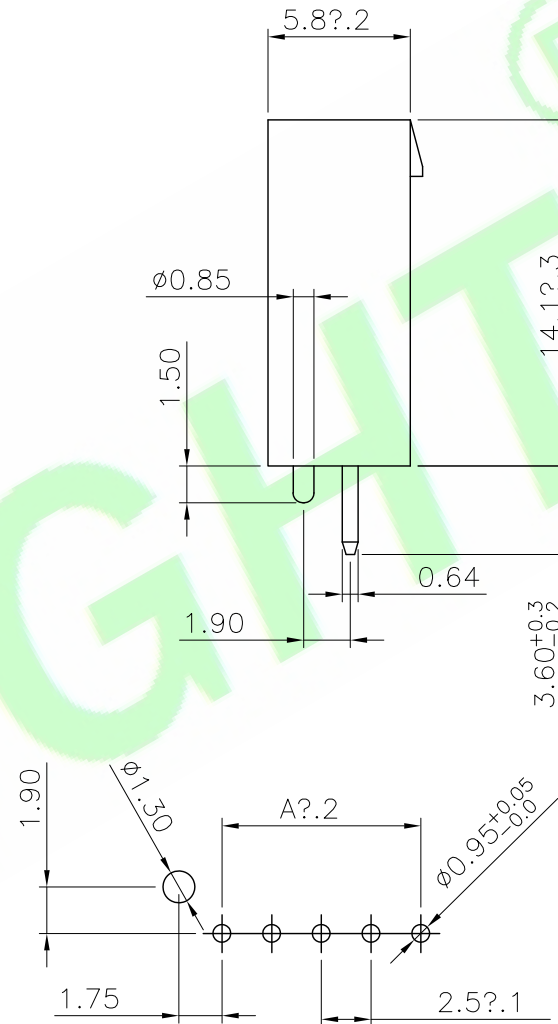
P.C.B LATOUT
