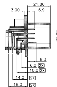
剖面 A-A
